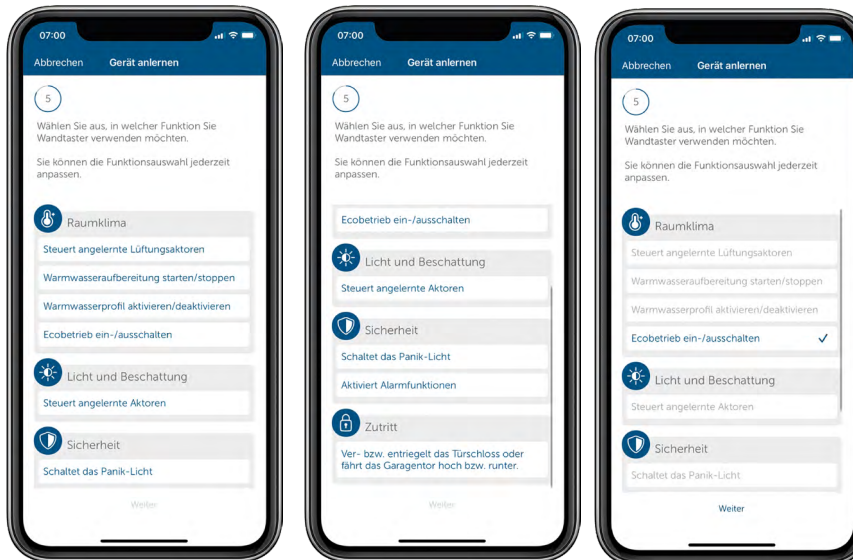
Abbildung 9: Screenshots Lösungszuweisung
