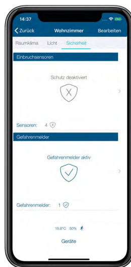
Abbildung 44: Sicherheitsinformationen Raumansicht
