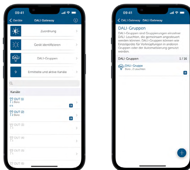
Abbildung 99: Screenshot DALI-Gruppen
