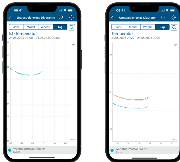
Abbildung 125: Screenshot Diagrammanzeige
