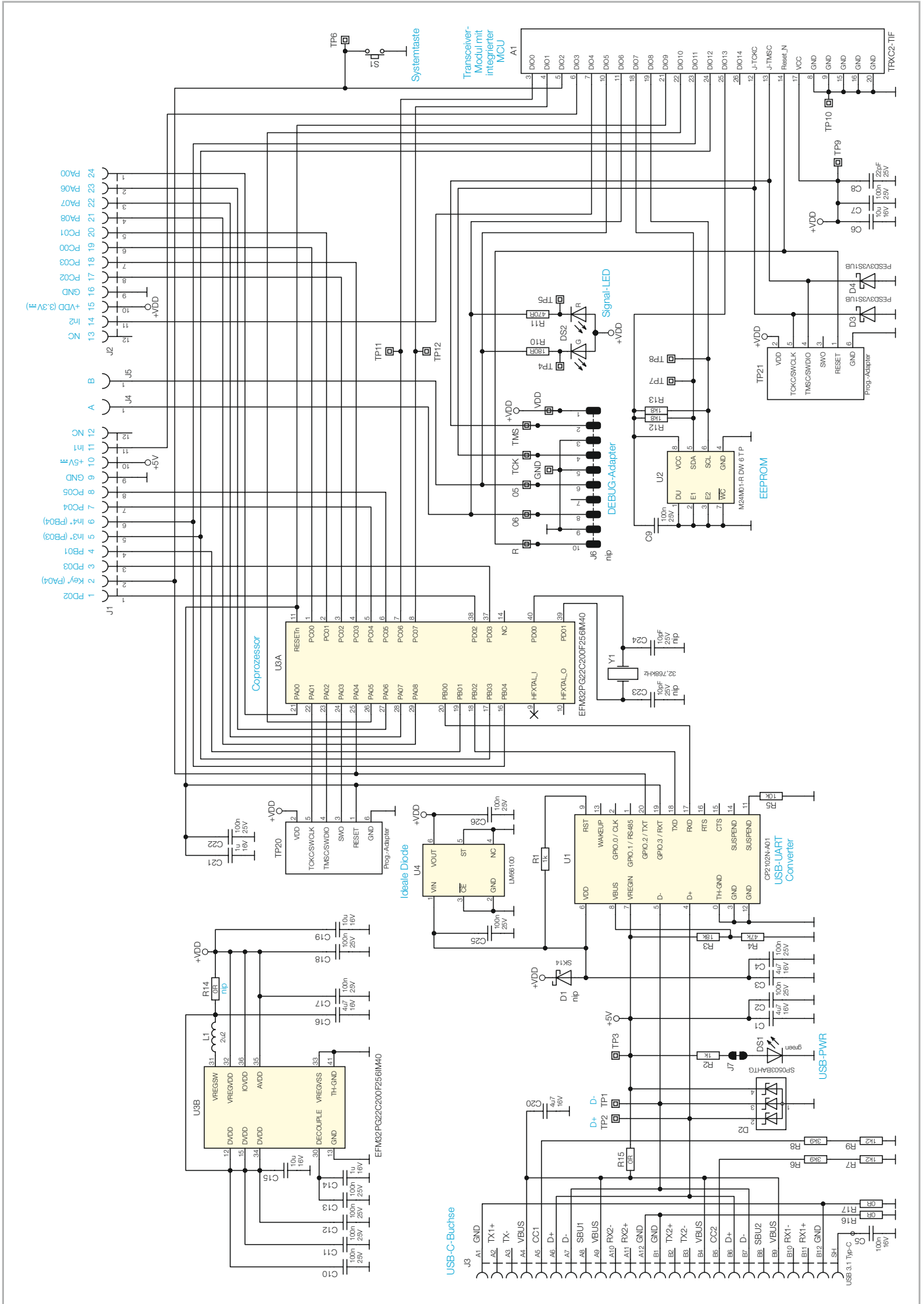
Bild 1: Schaltbild der Smart Home Sensor-Base
