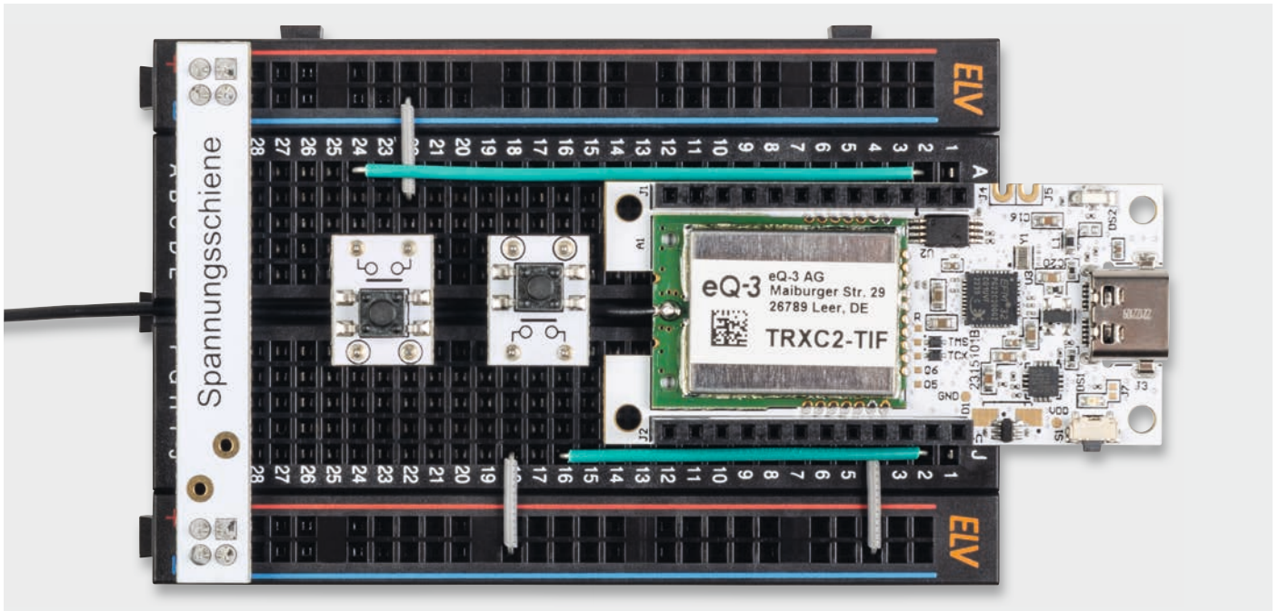
Bild 3: Breadboard-Aufbau als Tasterinterface
